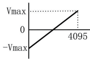
Fig. 2: Velocity linear mapping
