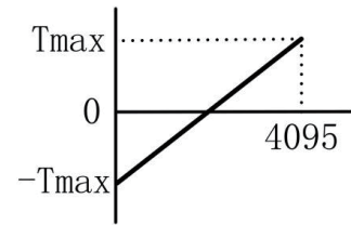
Fig. 3: Torque linear mapping
